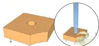
LFBJ-EMBETF Base angolare per tubo a bolle centrato e fibre ottiche
